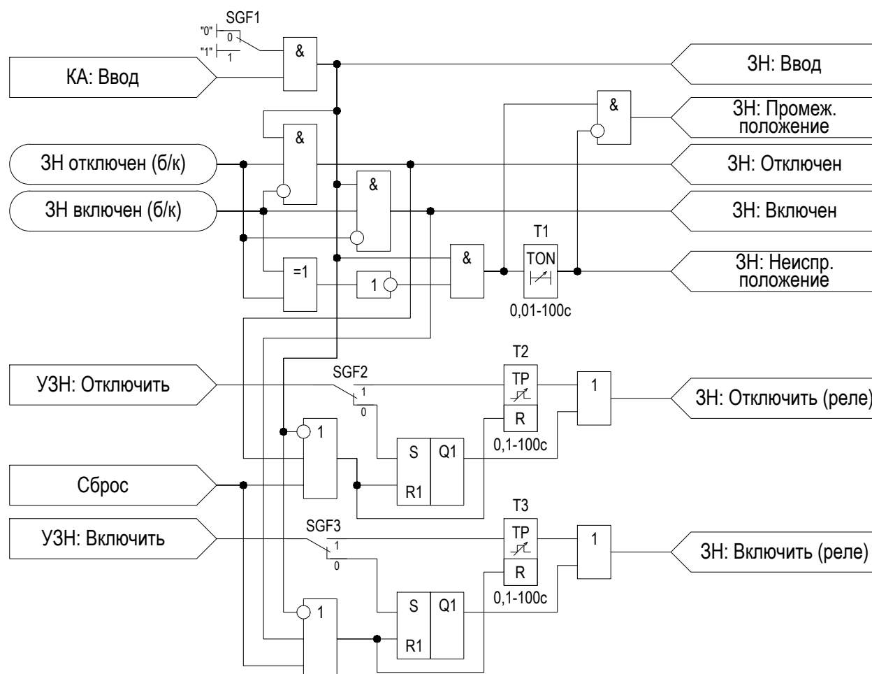
Рисунок 2.66 – Функциональная схема «3Н»
