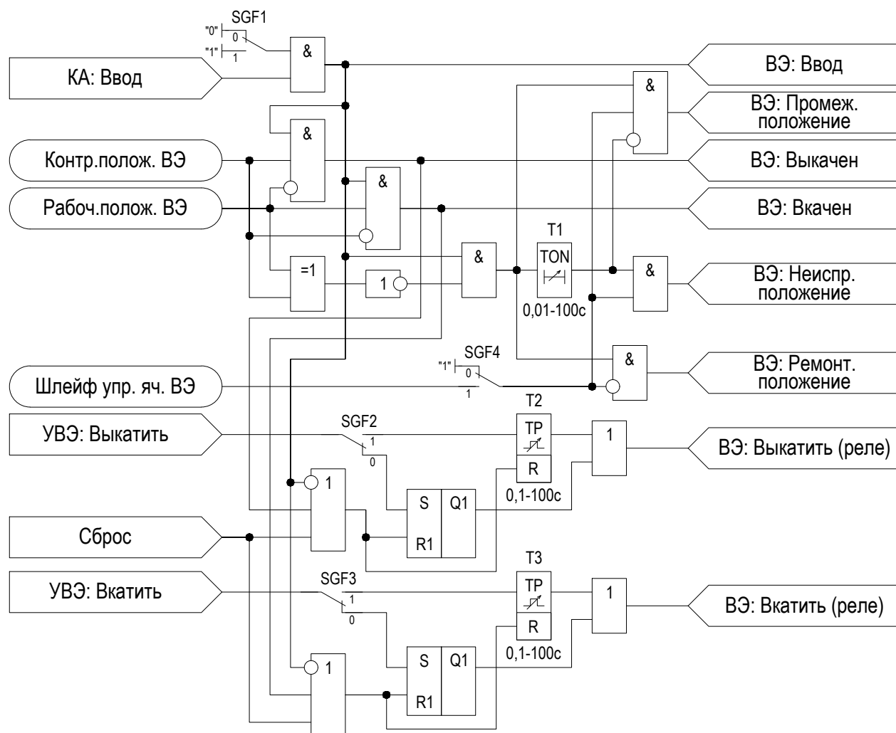
Рисунок 2.67 – Функциональная схема «ВЭ»
